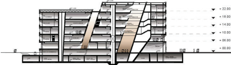
SCHNITT BB
