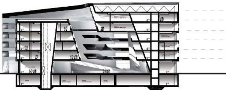
SCHNITT CC
