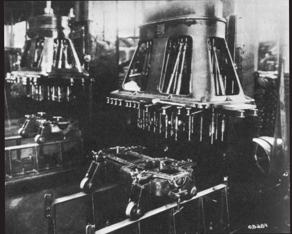
Πρόσδεση στροφαλοθάλαμου για διάτρηση, Highland Park, 1913.
