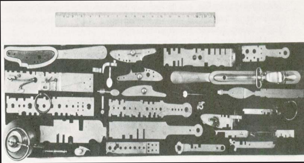
Ελεγκτήρες για τον έλεγχο έτοιμων κομματιών καραμπίνας (inspection gauges), Springfield armoury 1841.
