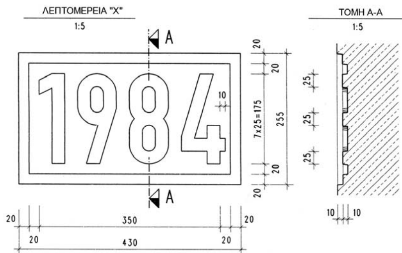
Σχήμα 4.3.7.8β
