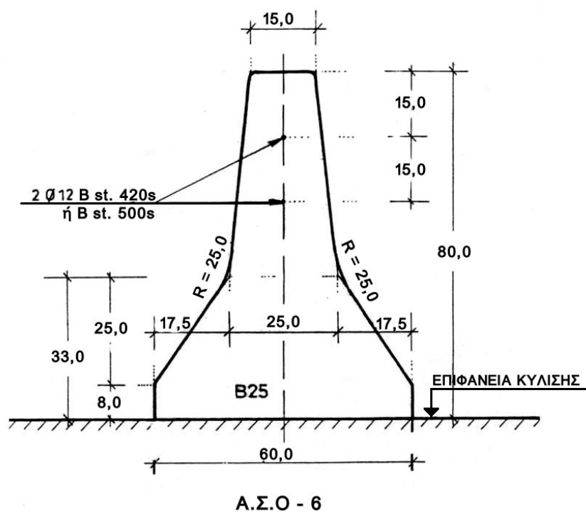
Σχήμα 4.3.1.20.(2)ιβ
