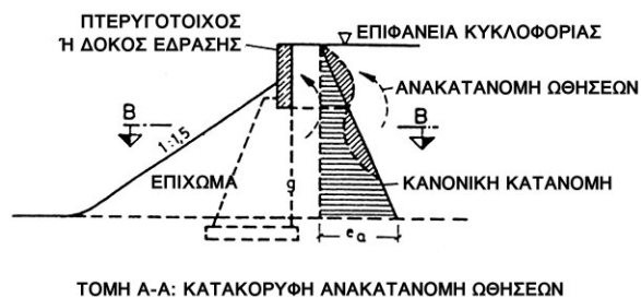
Σχήμα 4.3.7.3.(3)α
