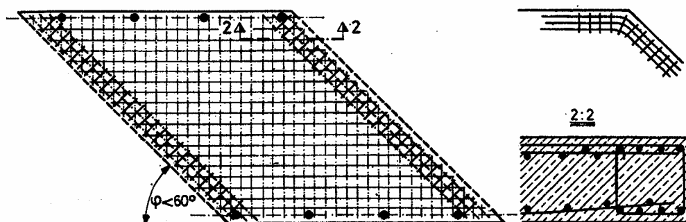
Διάταξη άνω και κάτω οπλισμού σε πλακογέφυρες με γωνία λοξότητος \varphi < 60^\circ
