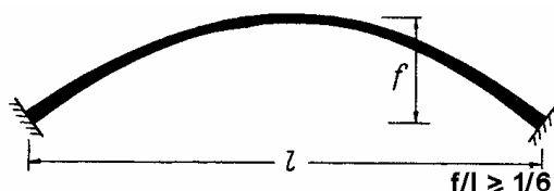
Σχήμα 4.3.4.(2).γ
