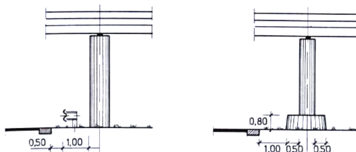
Σχήμα 2.5.3.(1).α.
