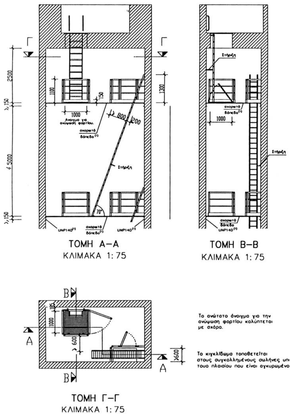
Σχήμα 4.3.8.(6)α
