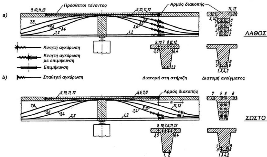
Σχήμα 4.3.1.10.(3)
