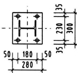
ΠΛΑΚΑ ΕΔΡΑΣΗΣ
