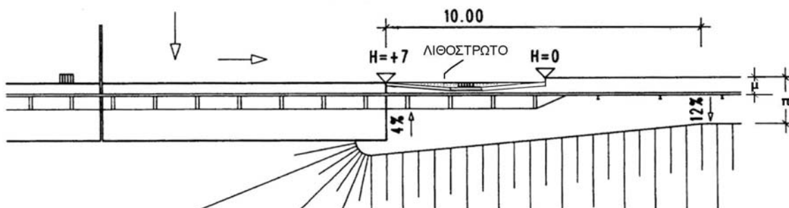
Σχήμα 4.3.7.7.(2)β
