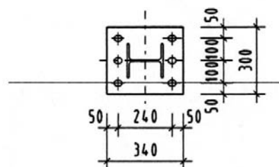
ΠΛΑΚΑ ΕΔΡΑΣΗΣ
