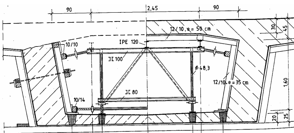
Σχήμα 4.3.3.2.(8)
