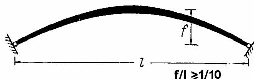
Σχήμα 4.3.4.(2).β
