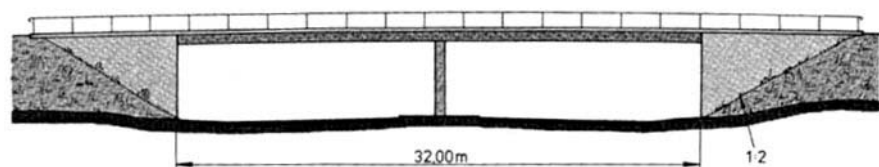
Σχήμα 4.1.12.(1)β
