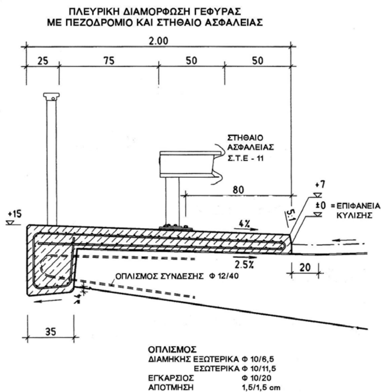
Σχήμα 4.3.1.15.(1)α
