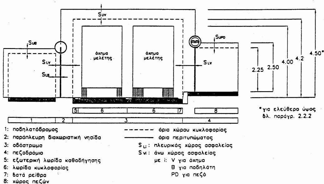
Σχήμα 4.1.9.(1)
