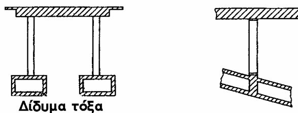
Σχήμα 4.3.4.(7).γ
