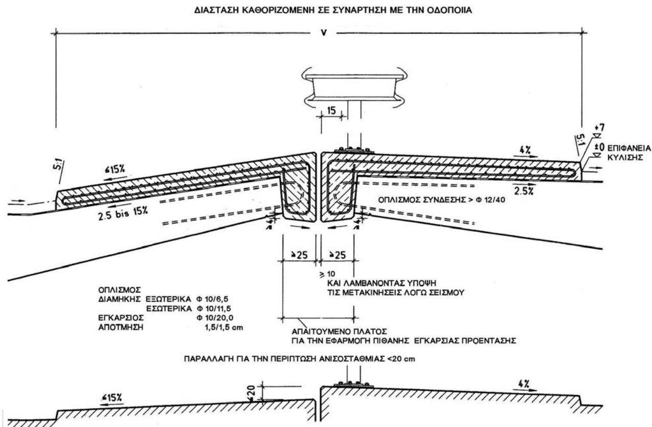
Σχήμα 4.3.1.16.(2)β
