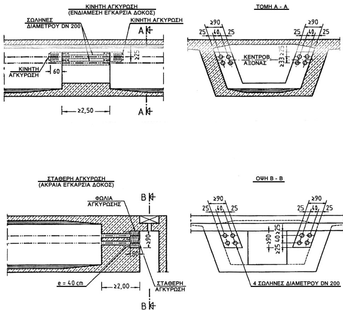
Σχήμα 4.4.1.(1)α
