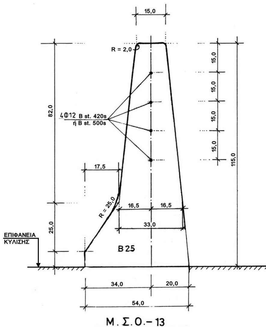
Σχήμα 4.3.1.20.(2)ια
