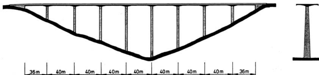
Σχήμα 4.3.8.(3).α
