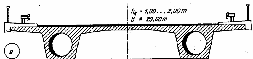
Δίδυμη πλακοδοκός
