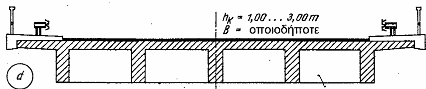
Εσχάρα δοκών
